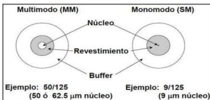
Figura N1 Tipos de fibra Óptica
