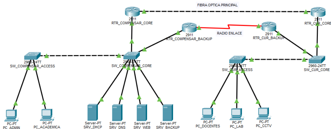
Figura N21 Montaje de conexión entre la infraestructura de la fundación universitaria compensar y la c.u.r compensa
